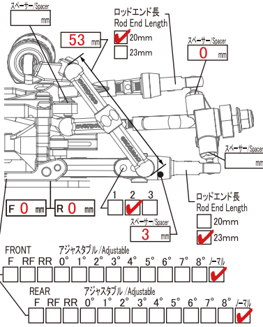
アジャスタブルアルミフロントサスペンションType-2 (Option) Adjustable Aluminum Front Suspension Arm Type-2
