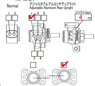
ショック / Shock: ノーマル / Normal ハイグレード / High Grade
