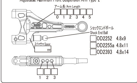
アジャスタブルアルミフロントサスペンションType-2 (Option) Adjustable Aluminum Front Suspension Arm Type-2
