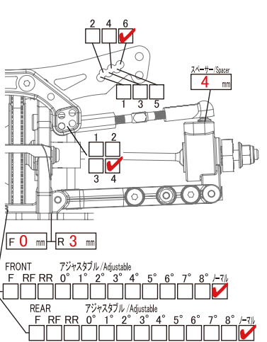
アジャスタブルアルミリアサスペンションType-2 (Option) Adjustable Aluminum Rear Suspension Arm Type-2
