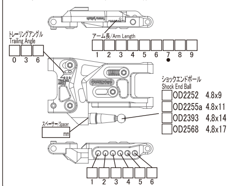
アジャスタブルアルミリアサスペンションType-2 (Option) Adjustable Aluminum Rear Suspension Arm Type-2
