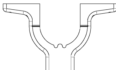
OD1471 ロアバルクヘッド(パープル) Lower Bulkhead (Purple)
