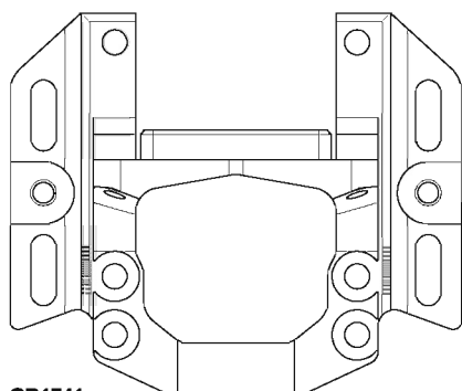
OD1741 フロントアッパーバルクヘッド Front Upper Bulkhead
