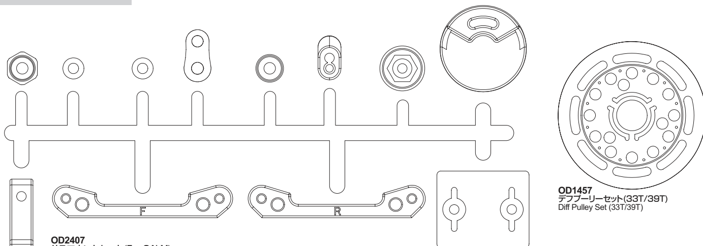
OD2407 サスマウントセット (For GALM) Suspension Mount Set (For GALM)
