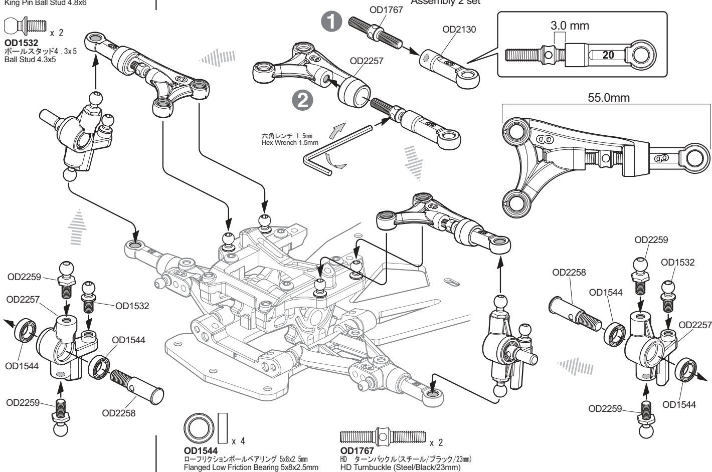
OD2259 キングピンボールスタッド4.8x6 King Pin Ball Stud 4.8x6
