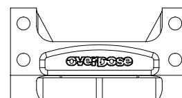
OD2311 アルミショックマウント Aluminum Shock Mount
