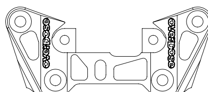
OD2305 アルミステアリングクラックマウント Aluminum Steering Crank Mount
