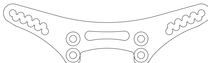
OD2304 フロントショックタワー (ブラック 3.0mm) Front Shock Tower (Black 3.0mm)
