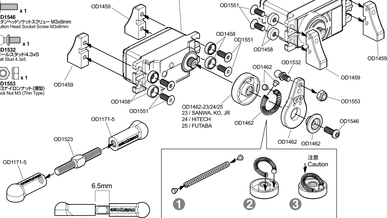
OD1551 フラットヘッドソケットスクリュー M3x8mm Flat Head Socket Screw M3x8mm
