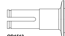
OD1513 ボールデフカップジョイント (POM/R) Ball Diff Cup Joint (POM/R)
