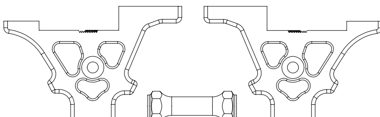
OD2314 アルミロアバルクヘッド L Aluminum Lower Bulk Head L
