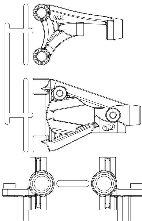
OD2257 フロントサスアーム&ナックルセット (For XEX spec.R, OD) Front Suspension Arm & Knuckle Set (For XEX spec.R, OD)
