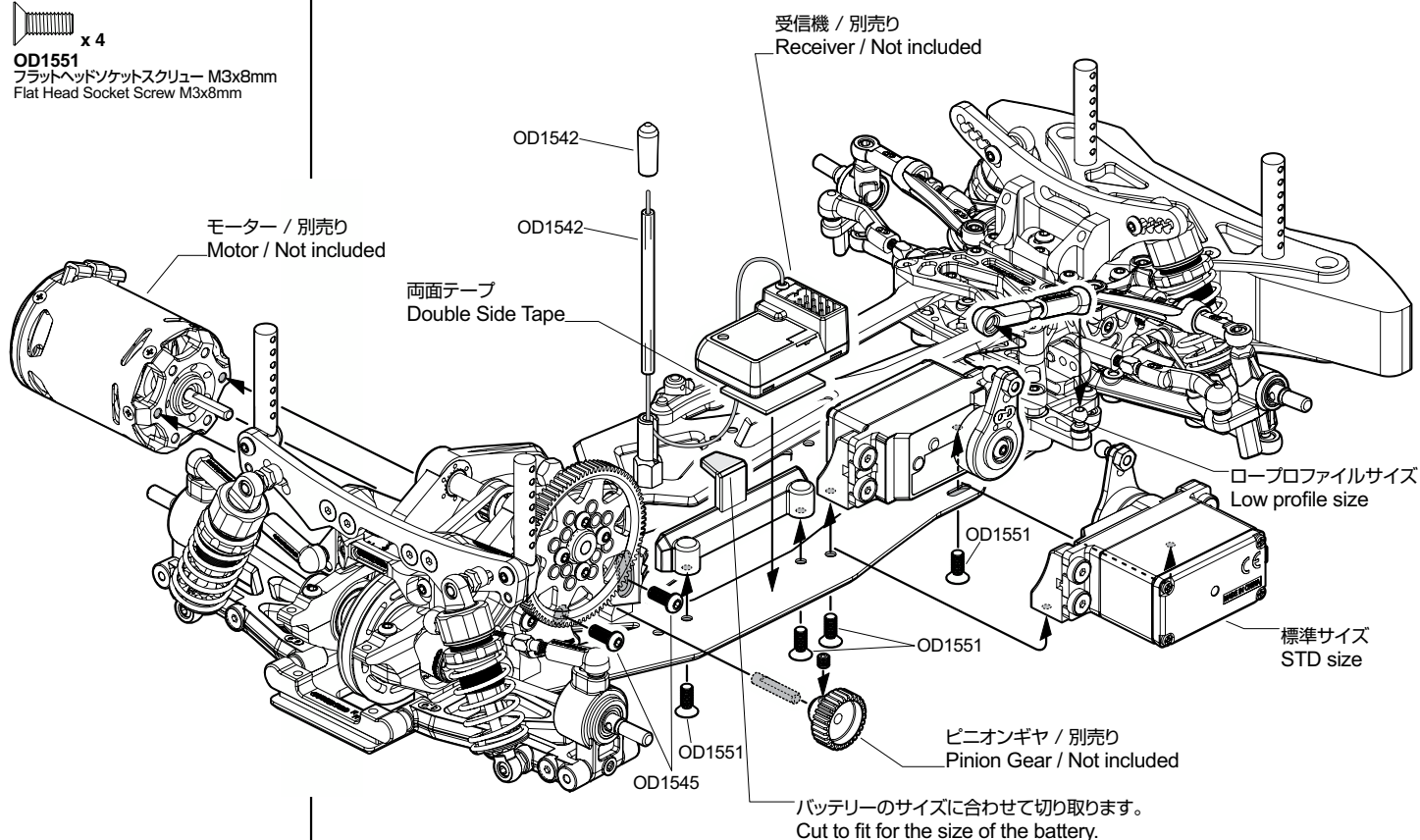
OD1545 ボタンヘッドソケットスクリュー M3x6mm Button Head Socket Screw M3x6mm
