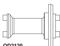
OD2120 リジッドアクスルボディ Rear Spool Axle Body
