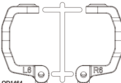
OD1464 C/ハブセット(6°) Hub Carrier Set (6 Degrees)
