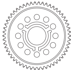
OD2104 デフファイナルギヤ 54T Differential Final Gear 54T
