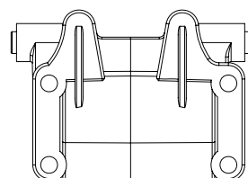
OD2130 ボールエンドセット (モリブデン) Ball End Set (Molybdenum)
