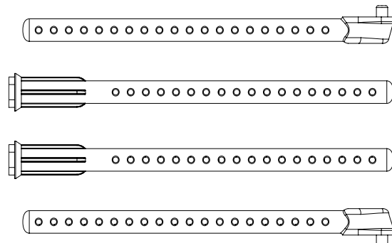
OD1461 ボディーポストセット Body Post Set
