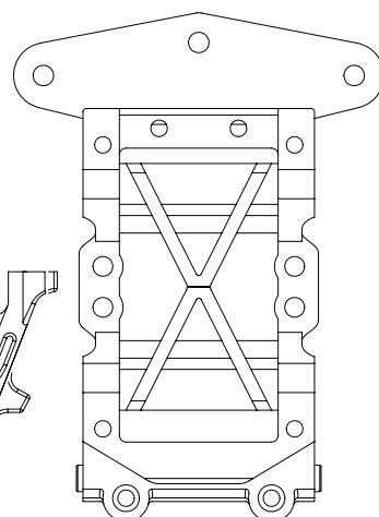
OD2256 フロントバルクヘッドセット (For XEX spec.R) Front Bulk Head Set (For XEX spec.R)
