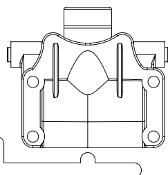
OD2103 リヤギヤケースセット Rear Gear Case Set
