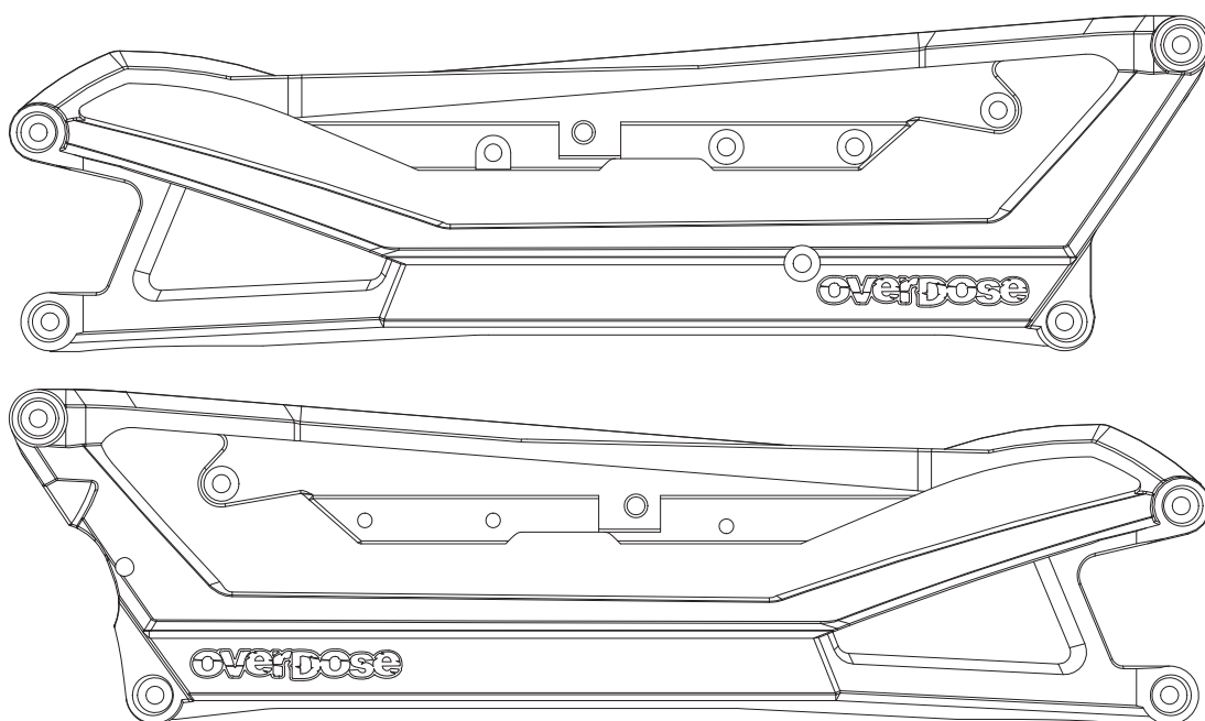
OD2102 メインフレームセット Main Frame Set
