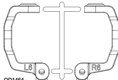
OD1464 Cハブセット(6°) Hub Carrier Set (6 Degrees)
